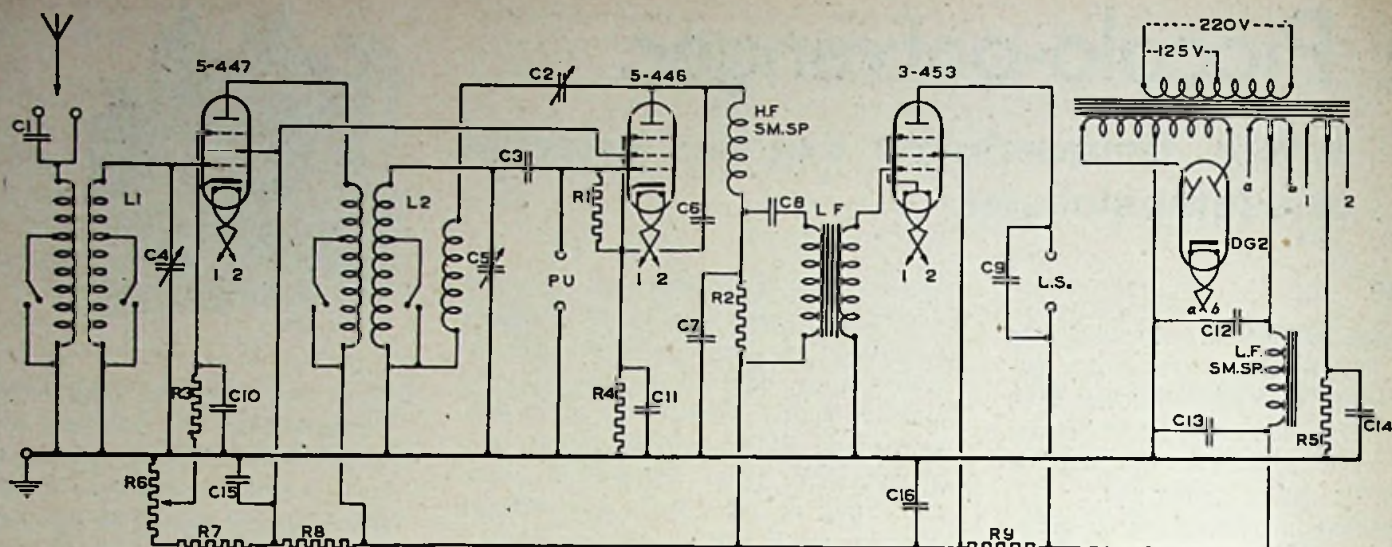
PRINCIPE SCHEMA
