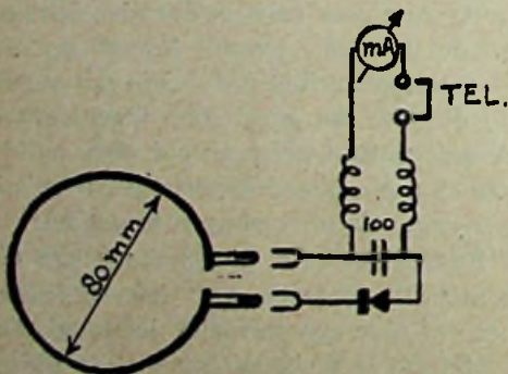
Fig. 1. Het schema van den indicator
