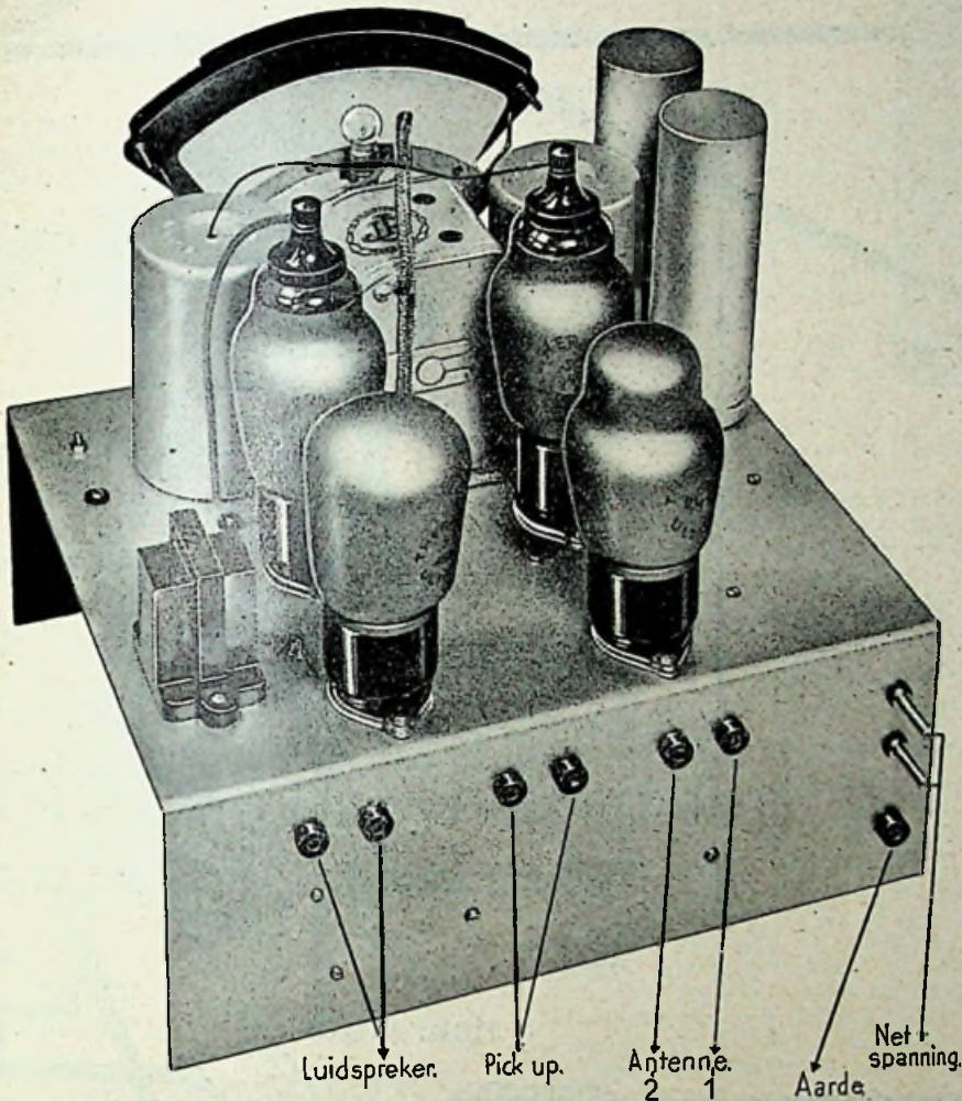
ACHTERZIJDE TOESTEL
